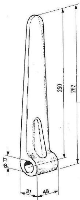
CERNIERA BILATERALE CORTA ZINCATA CON NERVATURA Cod. 09.0204 gr. 775
