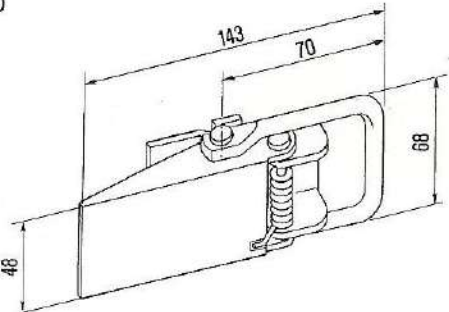
CHIUSURA A LACCIO Cod. 09.0826 gr. 350
