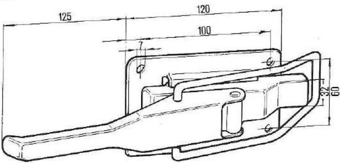
CHIUSURA TIPO VIBERTI Cod. 09.0822 gr. 950
