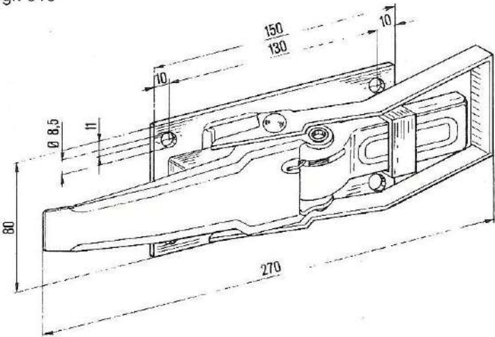
CHIUSURA TIPO TICO Cod. 09.0818 gr. 910
