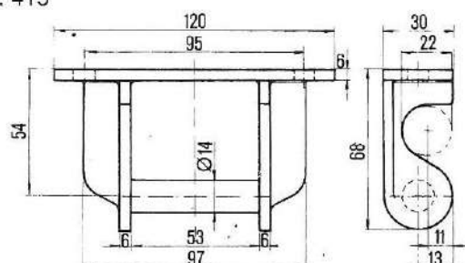
CERNIERA SPONDA ALLUM. PES. MM. 30 Cod. 09.0322 gr. 415
