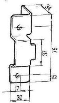
SCONTRINO TIPO VIBERTI Cod. 09.0824 gr. 105
