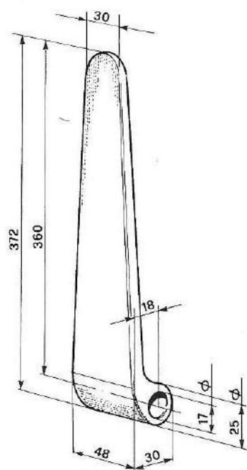
CERNIERA BILATERALE ALTA ZINCATA Cod. 09.0208 gr. 970
