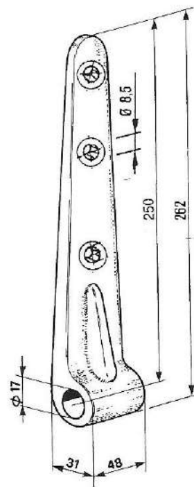
CERNIERA BILATERALE CORTA FORATA ZINCATA CON NERVATURA Cod. 09.0206
