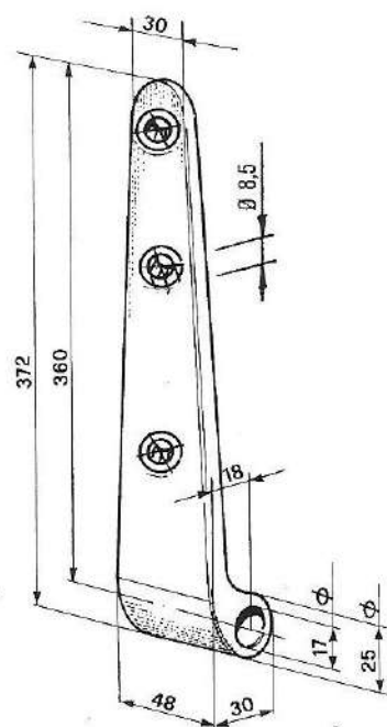
CERNIERA BILATERALE ALTA FORATA ZINCATA Cod. 09.0210
