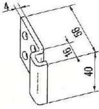
SCONTRINO A LACCIO Cod. 09.0828 gr. 85
