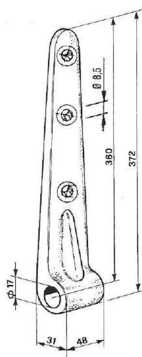
CERNIERA BILATERALE ALTA FORATA ZINCATA CON NERVATURA Cod. 09.0214
