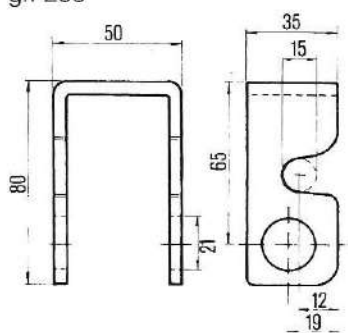
SUPPORTO GUIDA ASTA Cod. 09.0326 gr. 255
