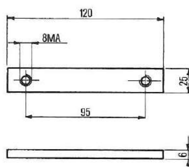
PIASTRINA INTER. 95 L. 25 Cod. 09.0318 gr. 150
