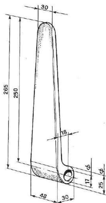
CERNIERA BILATERALE CORTA ZINCATA Cod. 09.0200 gr. 740
