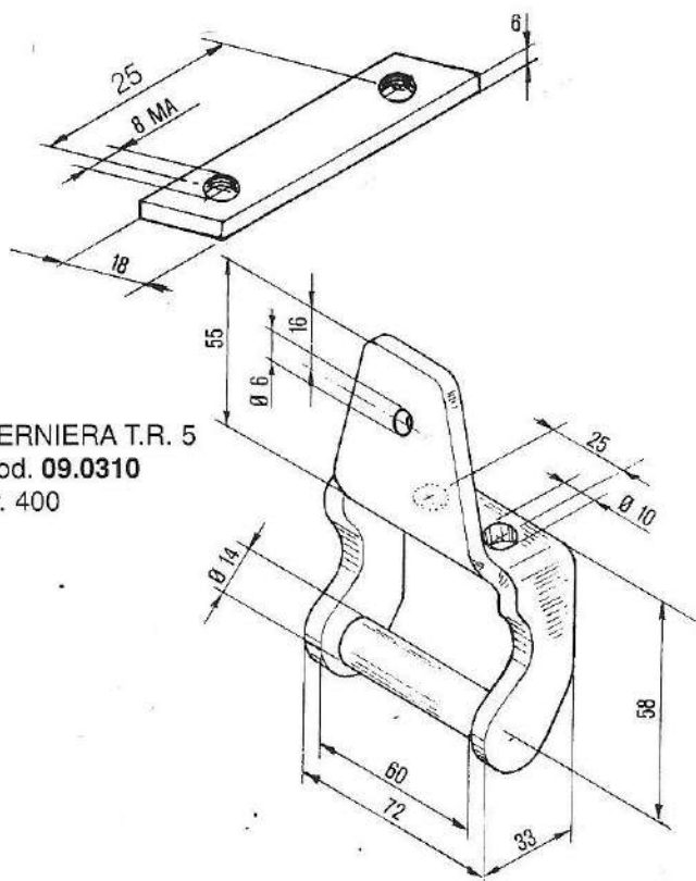
PIASTRINA INTERASSE 25 Cod. 09.0308 gr. 40
