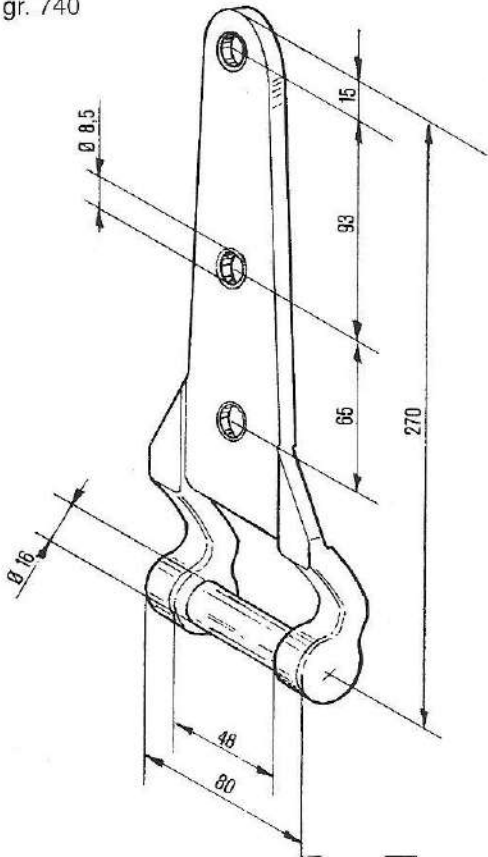
SUPPORTO GUIDA ASTA Ø 23 Cod. 09.0372
