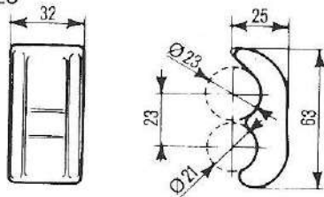
PALETTA Cod. 09.0376 gr. 125
