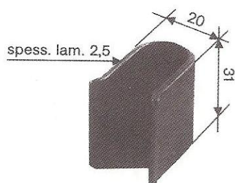
Cod. 08.0230 - Peso kg 0,040 Riscontro a piega aperta da saldare (versione grezzo)
