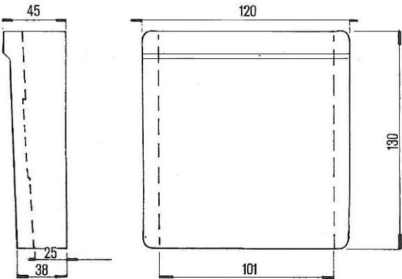
SEDE MONTANTE Cod. 08.0102
