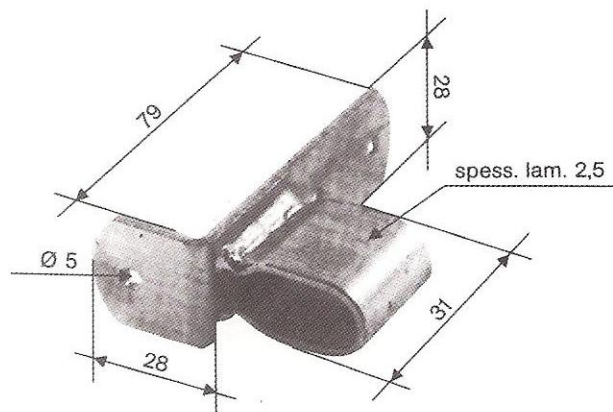
Cod. 08.0234 - Peso kg 0,100 Riscontro a squadra con fori da rivettare (zincato)
