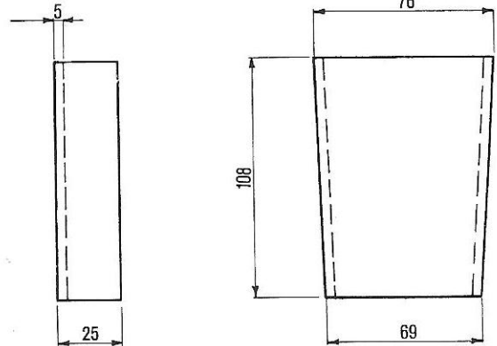
SEDE IN LAMIERA Cod. 08.0108
