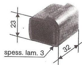
Cod. 08.0226 - Peso kg 0,080 Riscontro a piega chiusa da saldare (versione grezzo o zincato)
