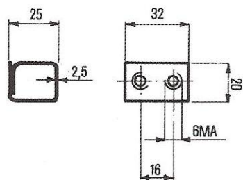
Cod. 08.0224 - Peso kg 0,050 Riscontro con fori filettati a piega chiusa da imbullonare (zincato)
