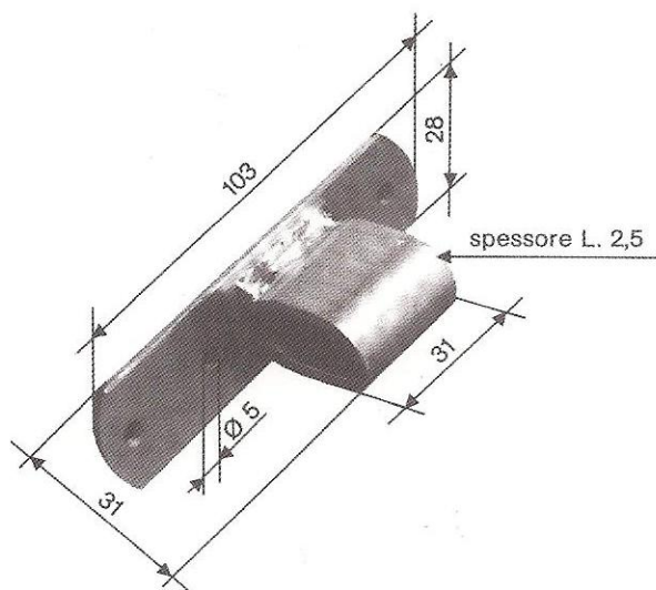
Cod. 08.0232 - Peso kg 0,100 Riscontro lineare da rivettare (zincato)
