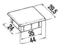
TAPPO PLASTICA Cod. 08.0228
