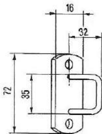
ANELLO TELONE Cod. 07.0412 gr. 35
