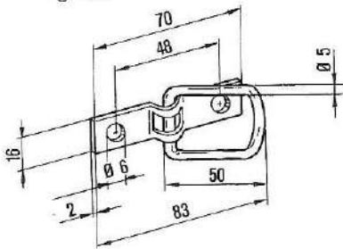
ANELLO TELONE Cod. 07.0404 gr. 30
