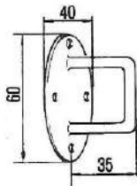
ANELLO TELONE Cod. 07.0418 gr. 37
