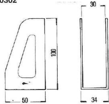
PIASTRINA PER SUPPORTO TIPO R. Cod. 07.0308 gr. 85
