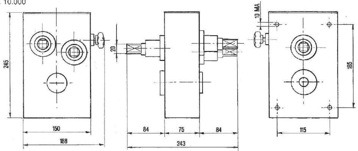
RIDUTTORE TIPO VR 1:8/1:16 Cod. 07.0104 gr. 10.000
