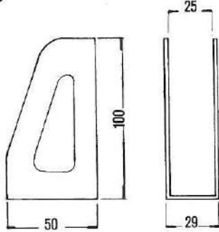
SUPPORTO ASTA CENTINA MM 25 TIPO R Cod. 07.0304
