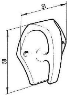
GANCIO TELONE TIPO COBRA NYLON GRIGIO Cod. 07.0400 gr. 15
