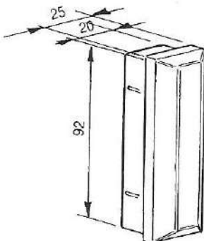
TAPPO ASTA CENTINA IN GOMMA Cod. 07.0314 gr. 100
