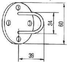
ANELLO TELONE Cod. 07.0420 gr. 37
