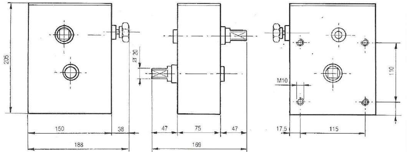
RIDUTTORE TIPO VR 1:8 Cod. 07.0102 gr. 6500
