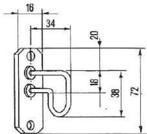
ANELLO TELONE Cod. 07.0414 gr. 38
