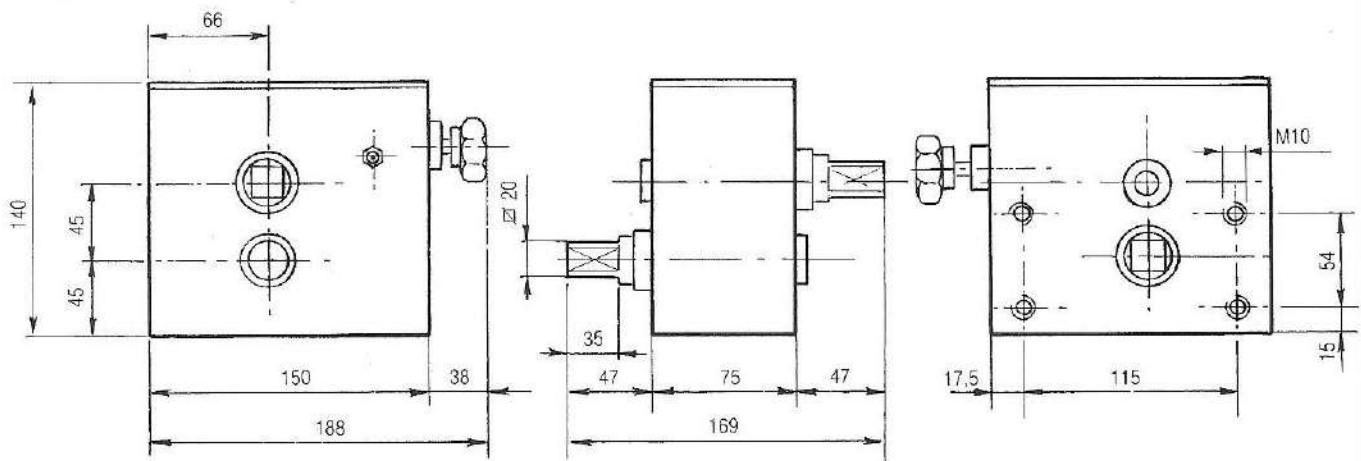
RIDUTTORE TIPO VR 1:4 Cod. 07.0100 gr. 4250
