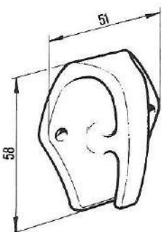
GANCIO TELONE TIPO COBRA NYLON BIANCO Cod. 07.0402
