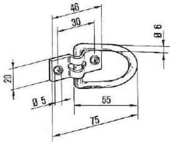
ANELLO TELONE Cod. 07.0406 gr. 35
