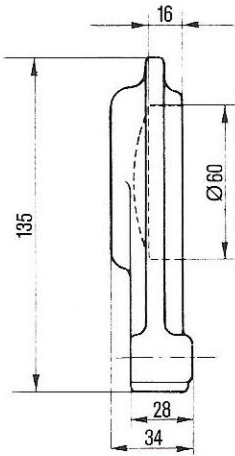
SUPPORTO VERRICELLO Ø 60 CON SALTARELLO Cod. 05.0216 gr. 1350
