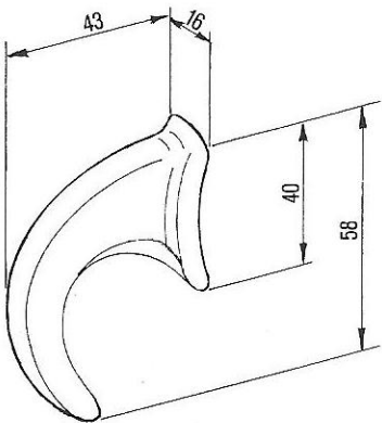
DENTE ELEFANTE PESANTE Cod. 05.0204 gr. 100
