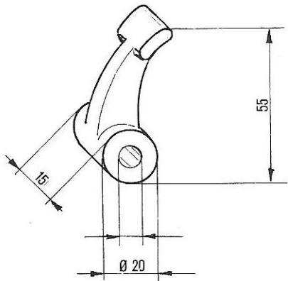
SALTARELLO LEGGERO Cod. 05.0206
