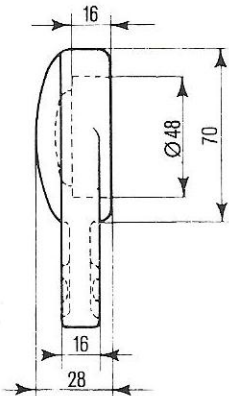
SUPPORTO VERRICELLO Ø 48 CON SALTARELLO Cod. 05.0212 gr. 865
