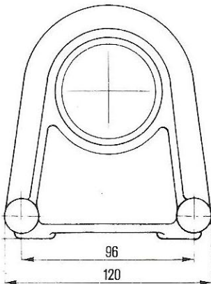
SUPPORTO VERRICELLO Ø 60 CON SALTARELLO Cod. 05.0216 gr. 1350
