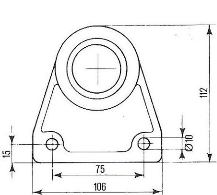
SUPPORTO VERRICELLO Ø 48 CON SALTARELLO Cod. 05.0212 gr. 865
