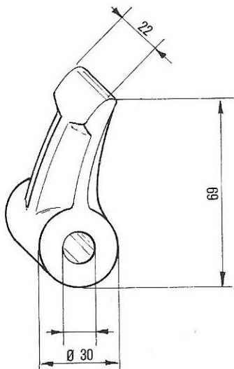
SALTARELLO PESANTE Cod. 05.0202
